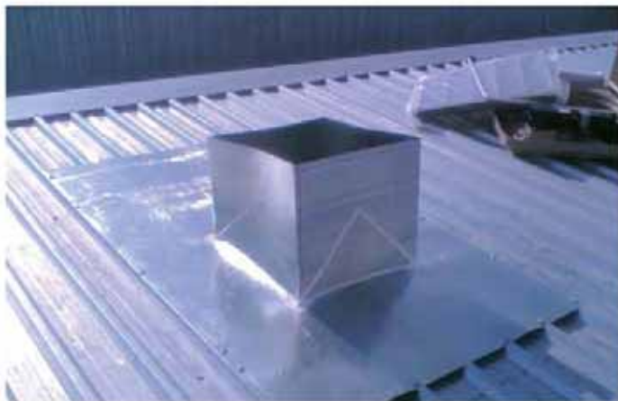
Sellado y fijación del vierteaguas al tejado
