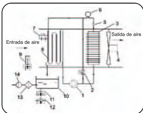
Esquema funcionamiento de los deshumidificadores
