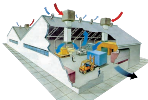
Esquema de instalación en naves industriales
