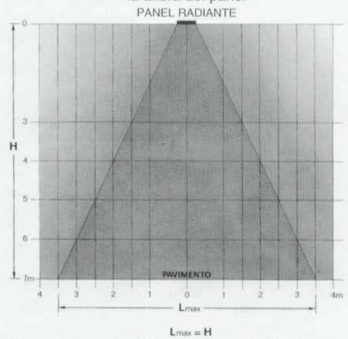
Gráfico de la zona de máxima radiación en función de la altura del panel
