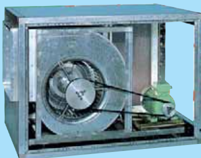
Serie EXCT con ventilador a transmisión por poleas
