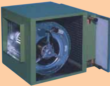
Aerotermos centrífugos TECNATHERM Serie AC para agua caliente ó con batería eléctrica.
