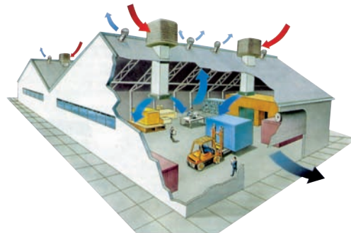
Esquema de instalación en naves industriales
